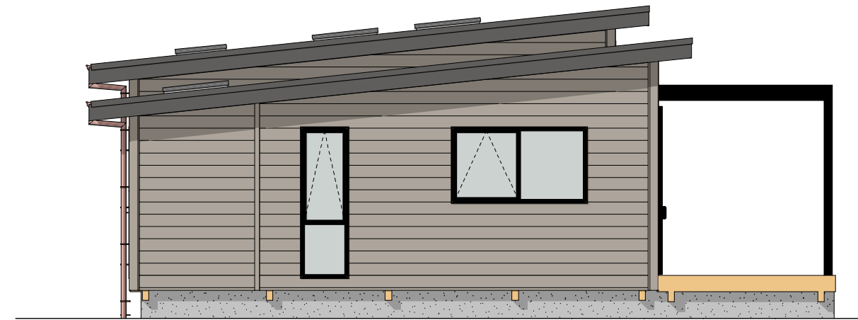
Elevation B 1:75
