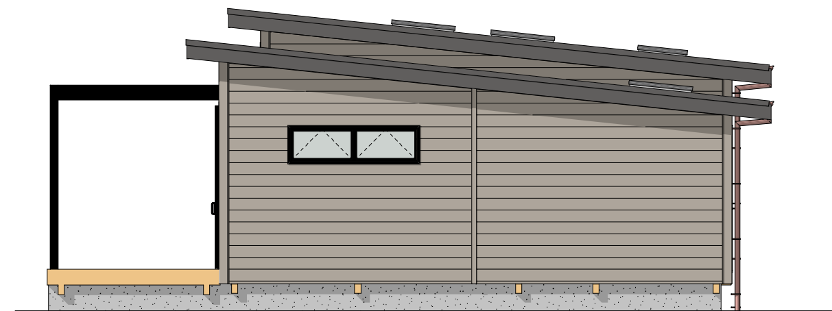
Elevation D 1:75
